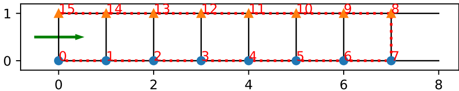
order='snakeFstyle'
