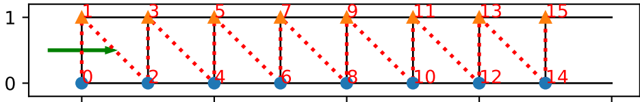
order='default'
